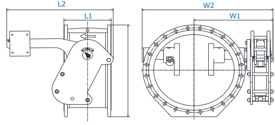
HİDROLİK DAMPERLİ KARŞI AĞIRLIKLİ TİLTİNG ÇEKVALF
