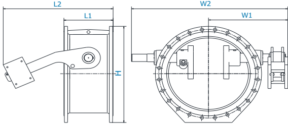
KARŞI AĞIRLIKLİ TİLTİNG ÇEKVALF
